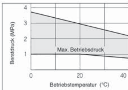
Berstdruck-Kurve
