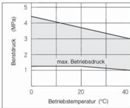
Berstdruck-Kurve
